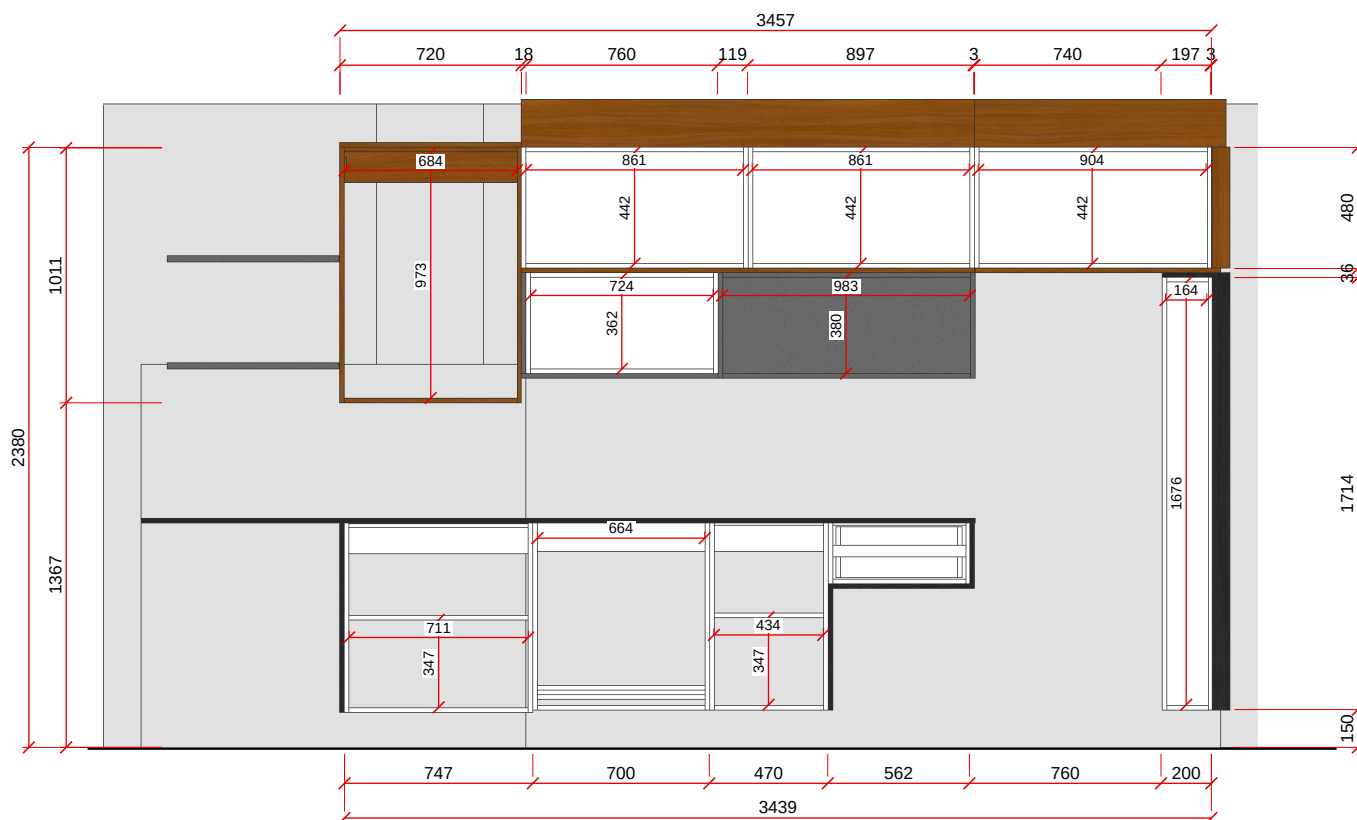
VISTA A - ESC. 1:30
