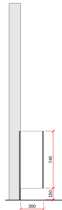
VISTA B - LATERAL - ESC. 1:25
