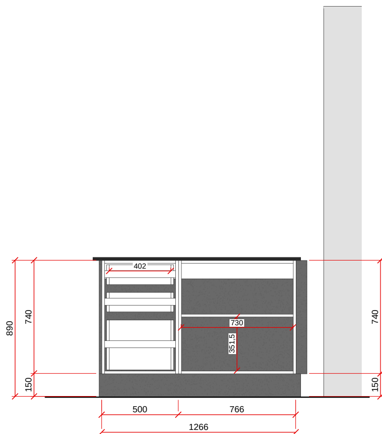
VISTA B - ESC. 1:25
