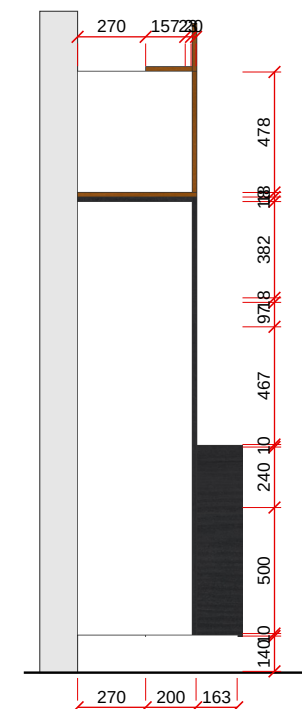
VISTA A - LATERAL - ESC. 1:30
